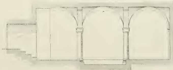
PRZEKROJ PO CDEF
